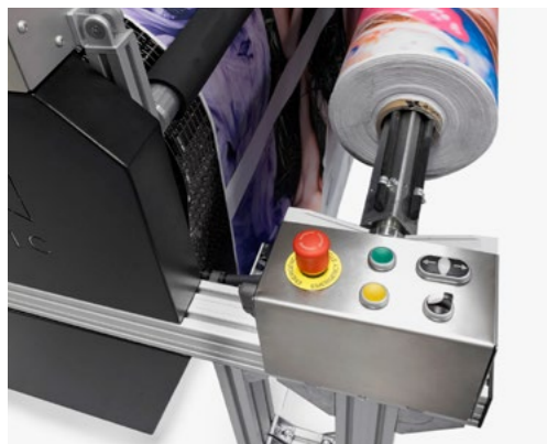
Automatic unwinding and edge control / Desbobinado y unidad de control del canto
